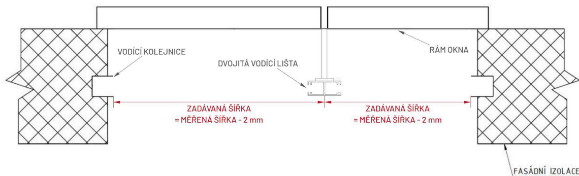
VRCHNÍ POHLED V ŘEZU PRO URČENÍ ŠÍŘKY DVOU A VÍCE ŽALUZIÍ NA HS PORTÁL A JINÉ DĚLENÉ PLOCHY
